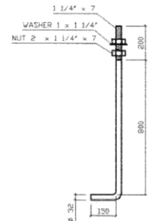
DET. ANCHOR BOLT
