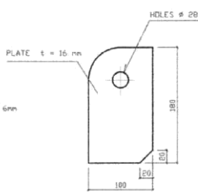
DET. RIP PLATE
