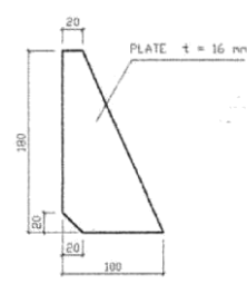
DET. RIP PLATE
